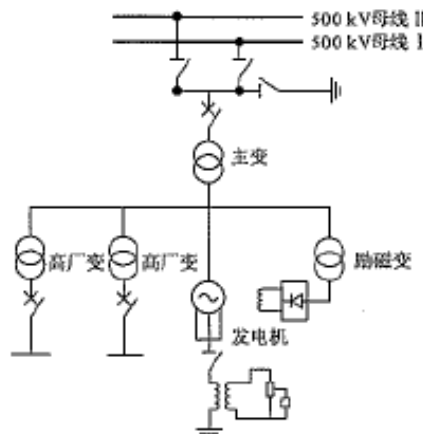
图 1 某电厂 1 000 MW 机组电气主接线图
