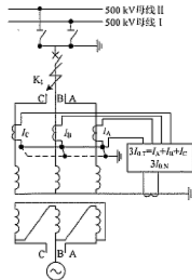
图 2 零序差动保护接线示意图
