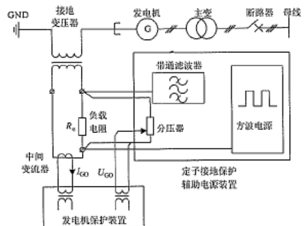
图 3 注入式定子接地保护示意图
