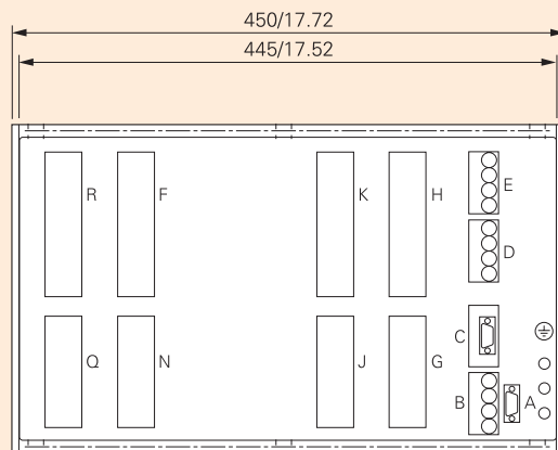
后视图3
