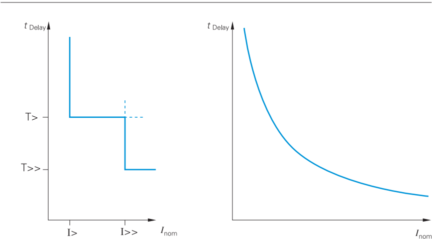
图 5/111：定时限过流保护
