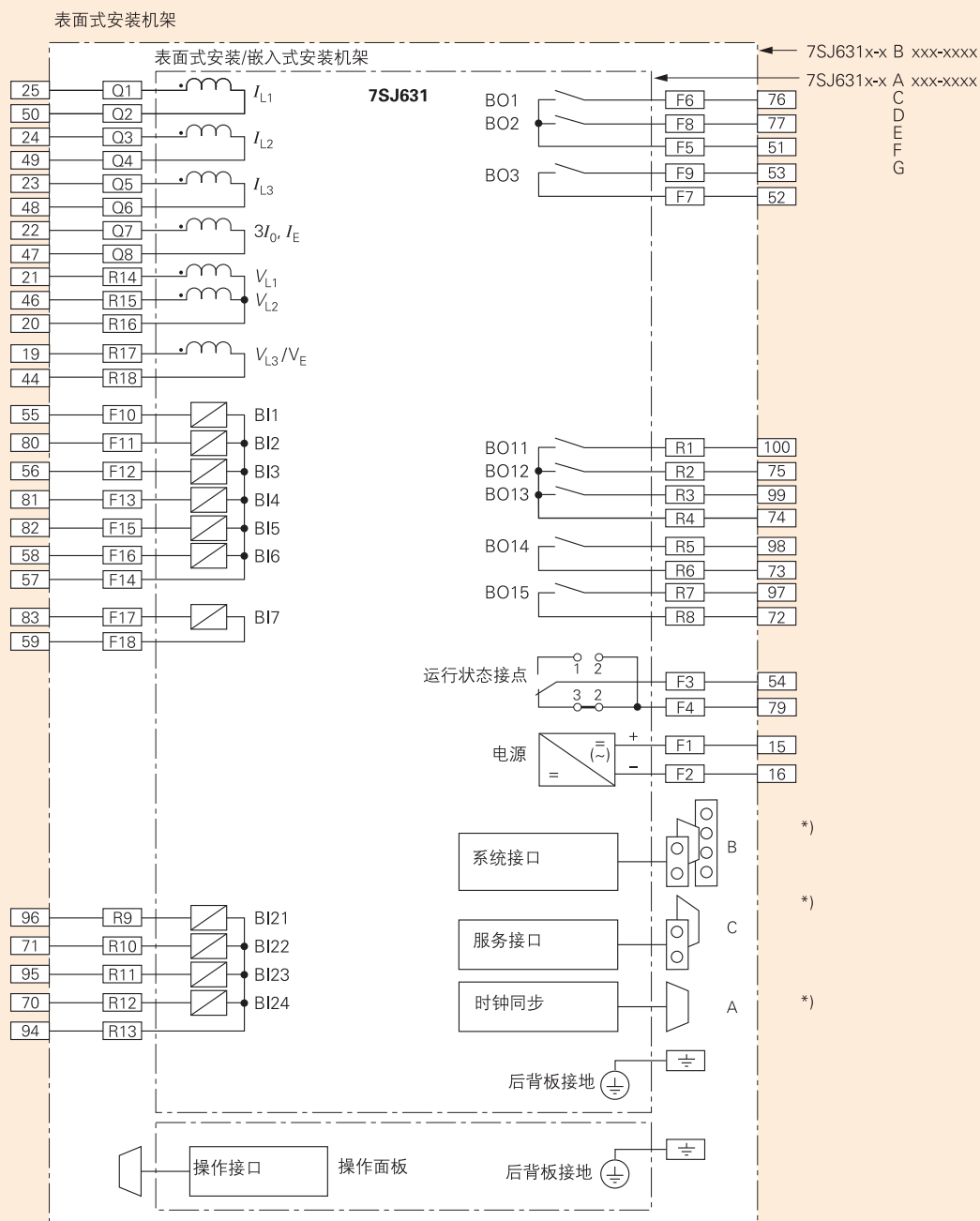
图5/137: 7SJ631接线图
