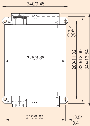
前视图
