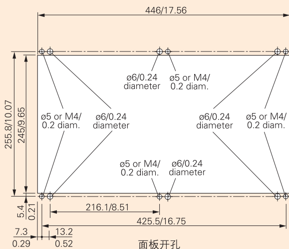
面板开孔
