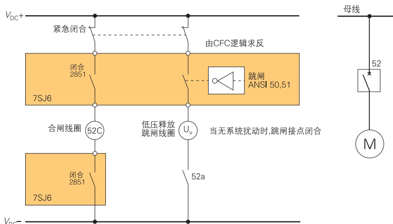
图5/134：带闭锁接点的欠压释放 (跳闸信号50取反)
