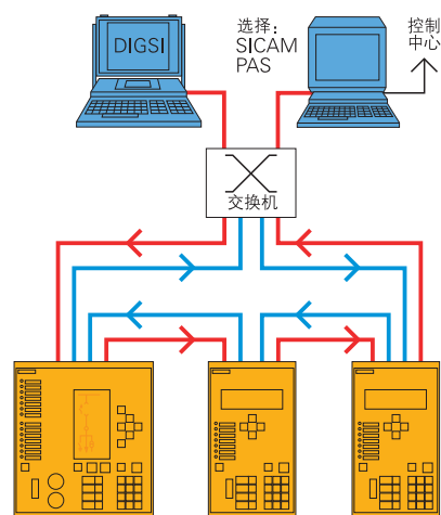
图5/124 由以太网、IEC 61850和光纤环网组成的站控总线
