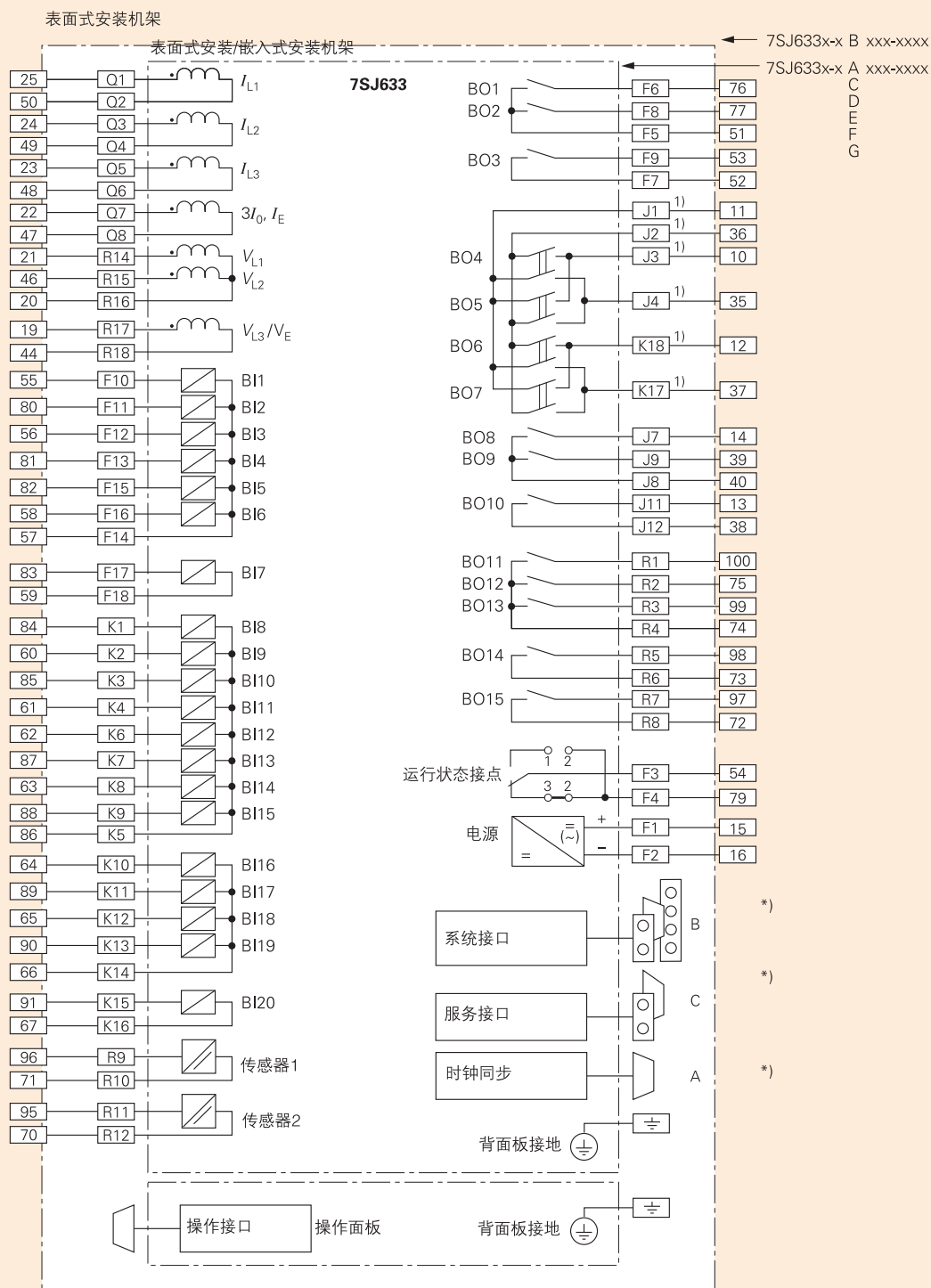
图5/139: 7SJ633接线图
