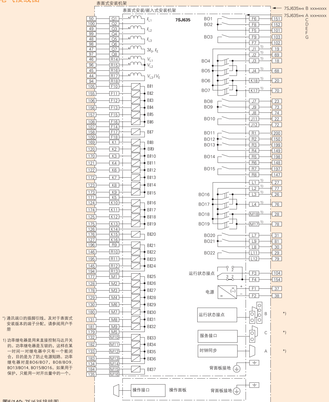
图5/140: 7SJ635接线图
