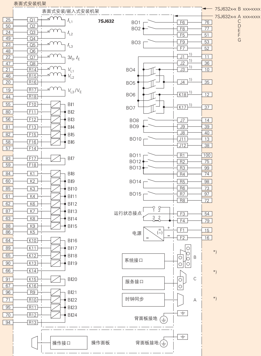
图5/138: 7SJ632接线图
