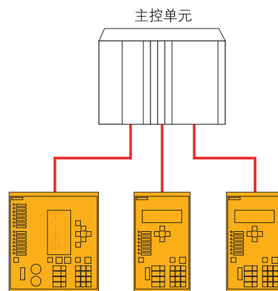
图5/122 IEC 60870-5-103：辐射形光纤连接
