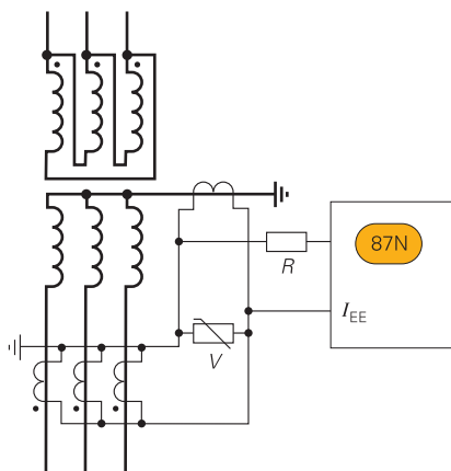
图 5/115: 高阻接地故障差动保护
