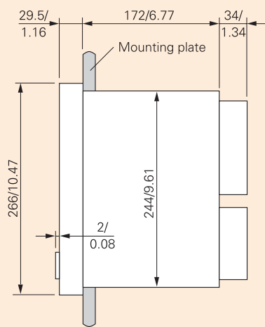
侧视图1
