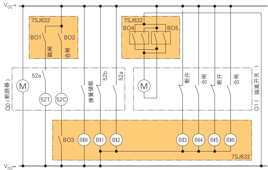
图5/118 7SJ632电机直接控制的典型接线图(没有熔丝的简化图) 开入量BO6和BO7是互锁的，这样同一时刻只能闭合二组接点
