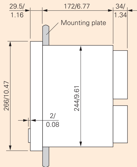
侧视图1
