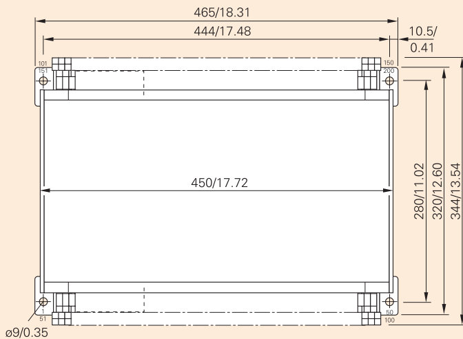
前视图
