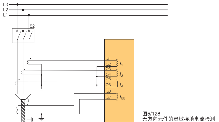
图5/127 无方向元件的残余电流回路
