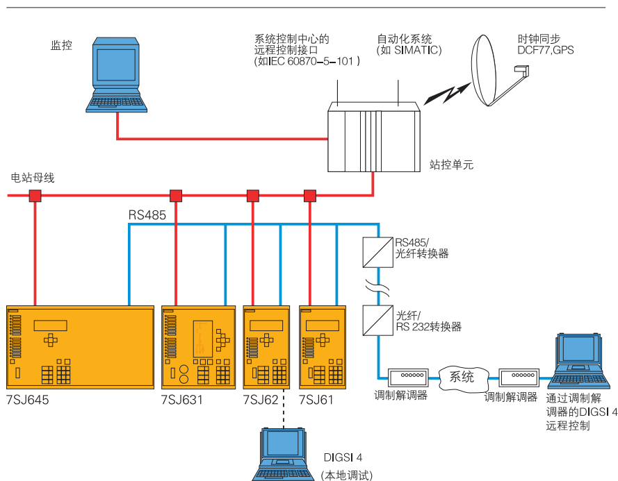
图5/125 系统解决方案/通讯
