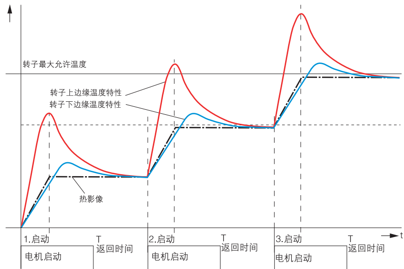
图 5/155: 重启抑制特性
