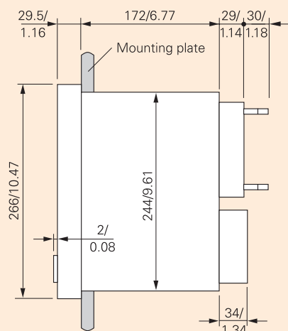
侧视图2
