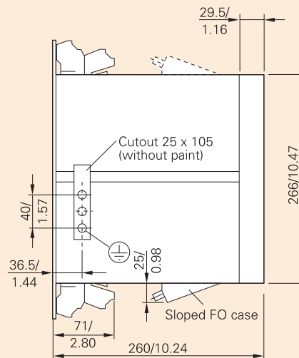
侧视图
