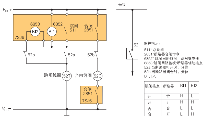
图5/135：带两个开入量的跳闸回路监视
