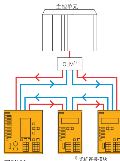
图5/123 PROFIBUS：光纤双环回路
