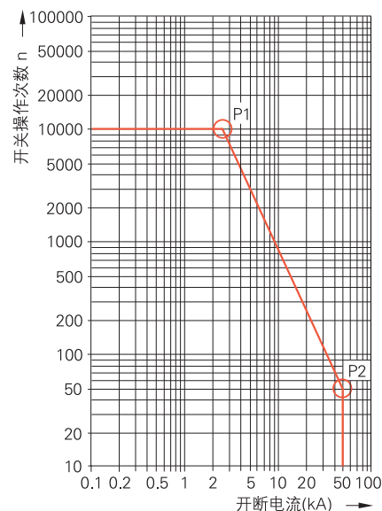
图 5/117: CB操作周期图表
