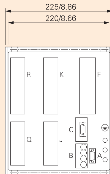
后视图 7SJ63
