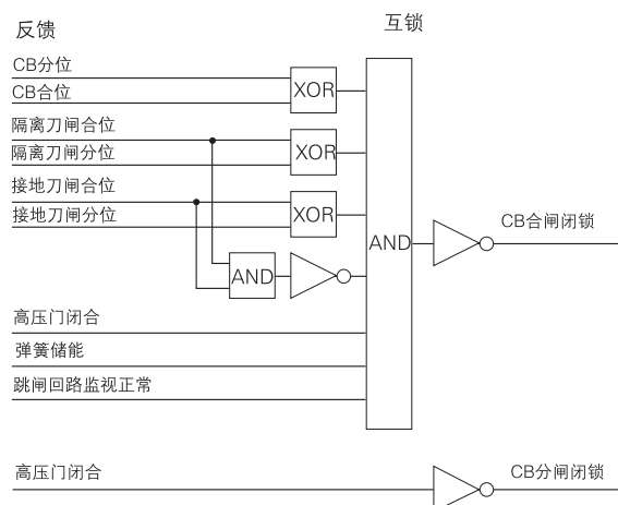
图5/120 示例：断路器互锁
