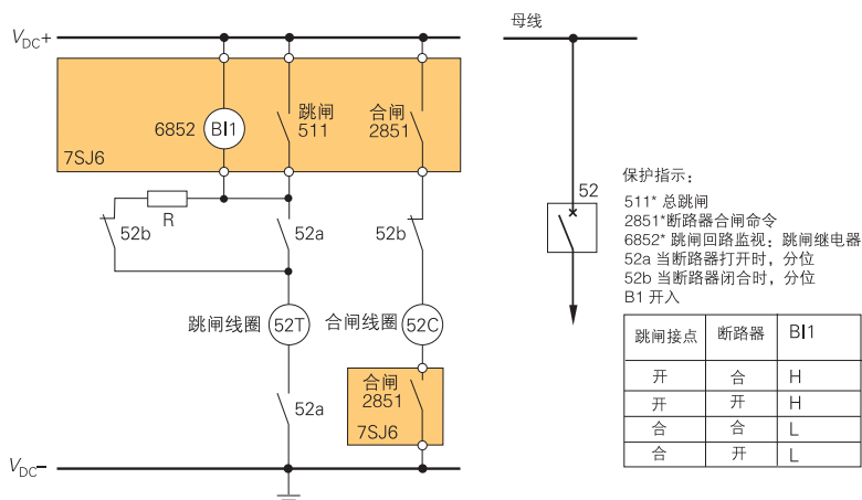
图5/136：带一个开入量的跳闸回路监视
