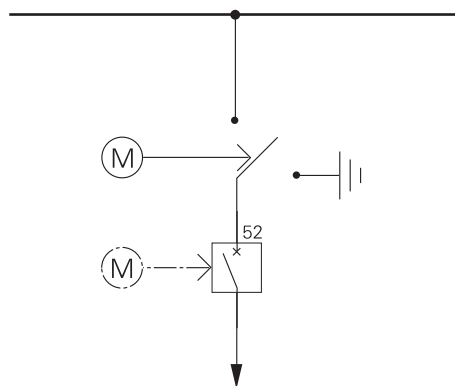
图5/119 示例：有断路器和电动机控制的三位置刀闸的单母线
