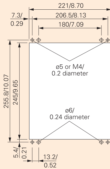
面板开孔
