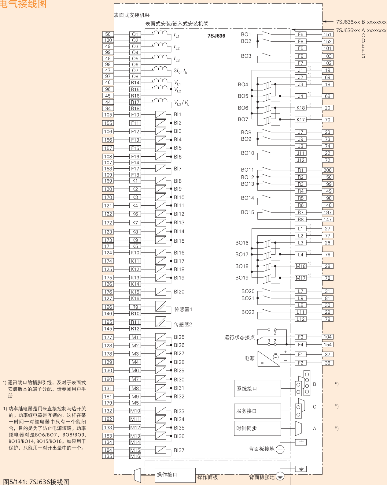
图5/141: 7SJ636接线图
