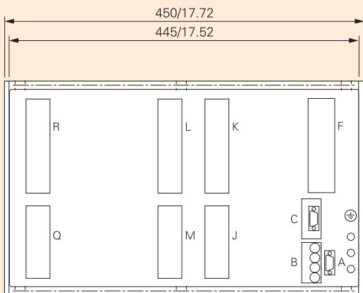
后视图2
